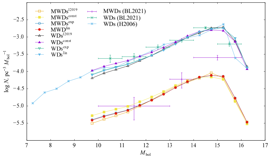
Рис. 2. Модельные ФС для всех БК и МБК — «WDs» и «MWDs» соответственно; Верхние индексы «const», «exp», «lin» и «12019» обозначают используемый нами в модели темп звездообразования — постоянный, с экспоненциальным или линейным спадом и темп звездообразования согласно Isern (2019) соответственно. Для сравнения представлены наблюдаемые ФС для известных БК в окрестности Солнца радиусом 250 пк (H2006) и для всех БК и МБК в объеме, ограниченном 20 пк (BL2021).
