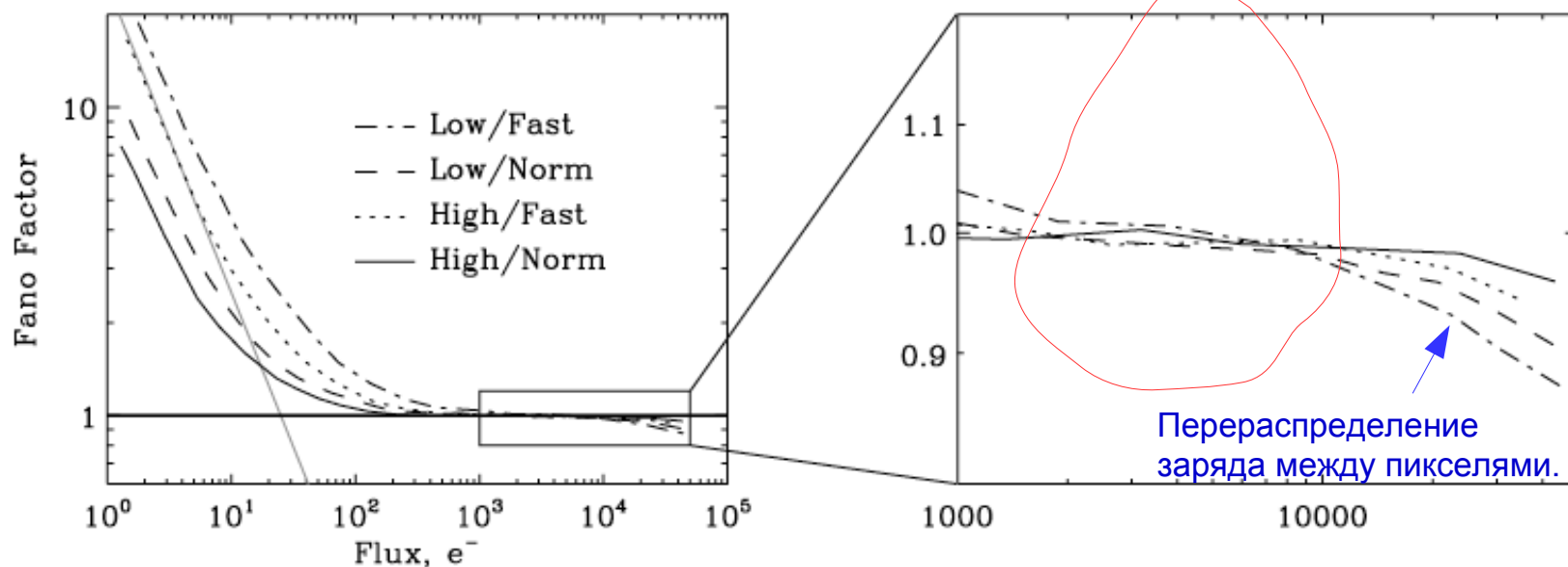
Рис. 1. Зависимость фактора Фано в изображении плоского поля от среднего потока для различных режимов работы тракта регистрации CCD42-90: Low и High — значения gain , равные 1.82e^-/\text{ADU} и 0.48e^-/\text{ADU} соответственно, а
